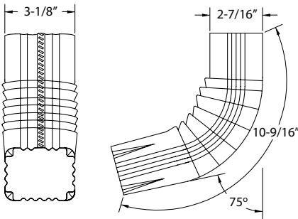
AAE23 A-Elbow
