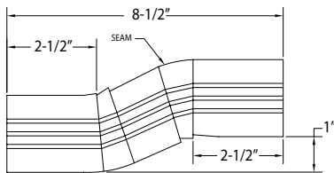
ABO1134A A-Offset
