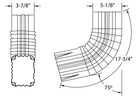
ABE245 B-Elbow
